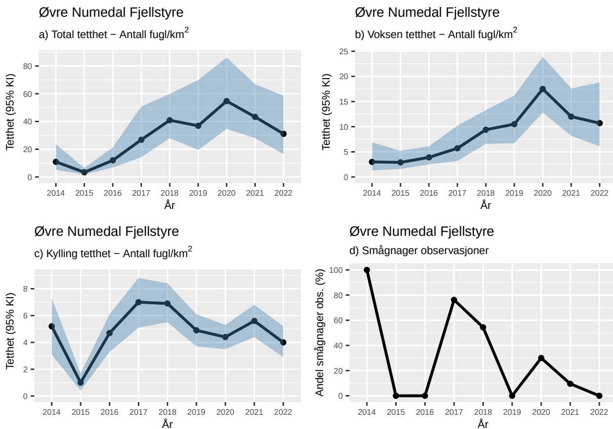
Figur 1. Figuren viser a) estimert total tetthet (antall observasjoner / km 2 ) for lirype, b) estimert voksen tetthet (antall voksne fugler observert / km 2 ) for lirype, c) estimert kylling tetthet (antall kyllinger observert / km 2 ) for lirype og til slutt d) antall linjer med sett smågnagere / antall takserte linjer. Det blå feltet rundt trendlinjen i figur a), b) og c) representerer 95% konfidensintervallet til estimatet.
